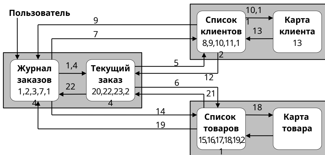
Рисунок 1.1 – Схема навигации
